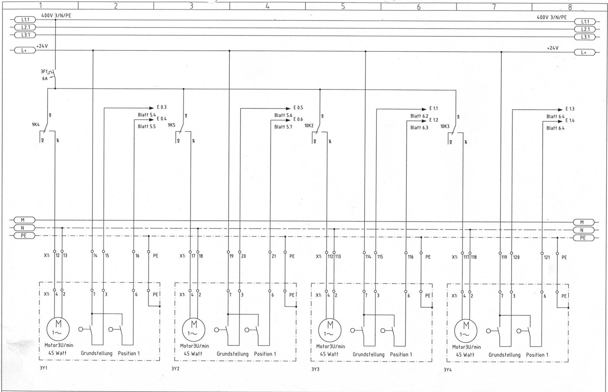
Umschaltweiche 1 (oben)
