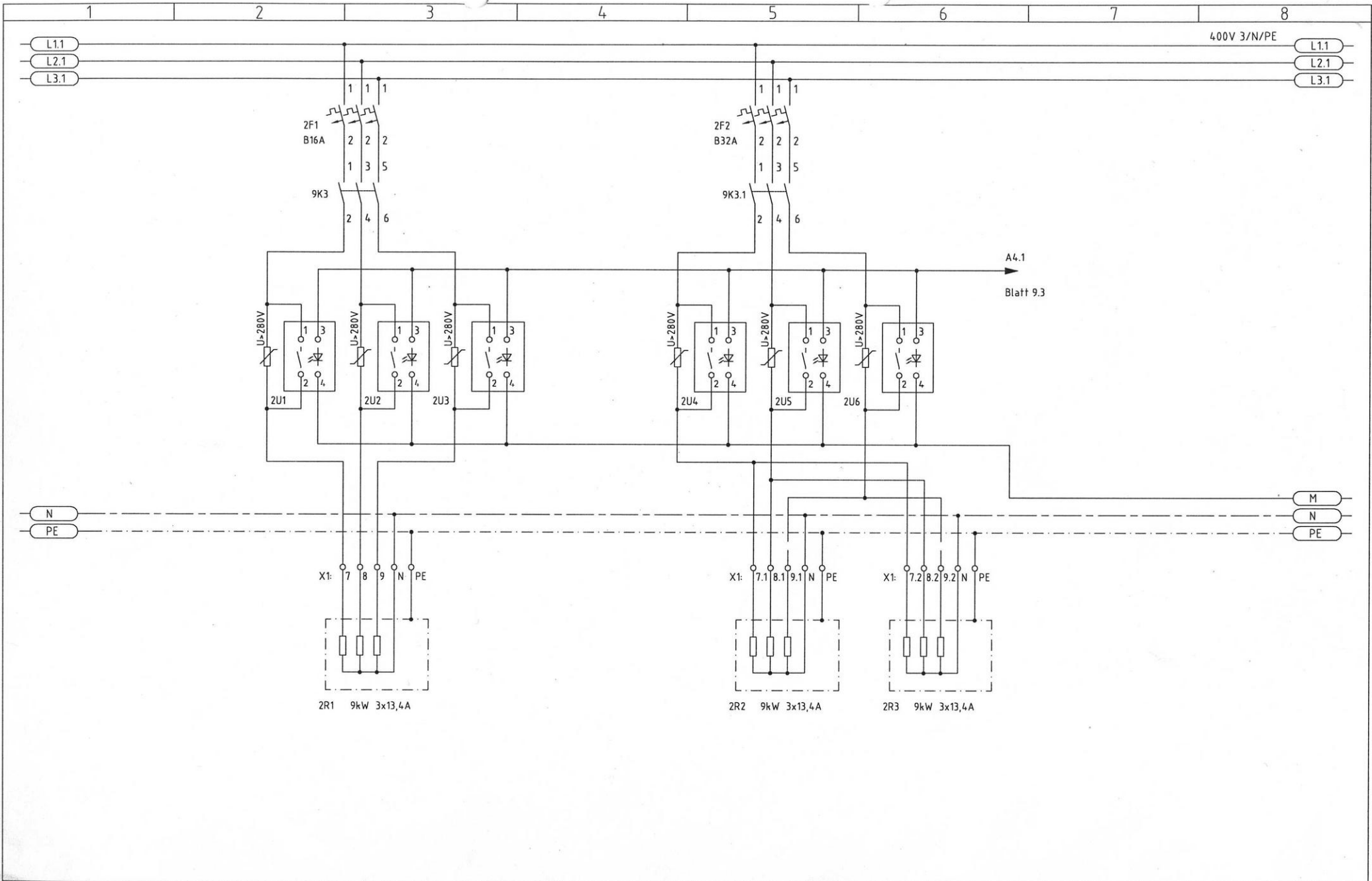
Regenerierheizung 1
