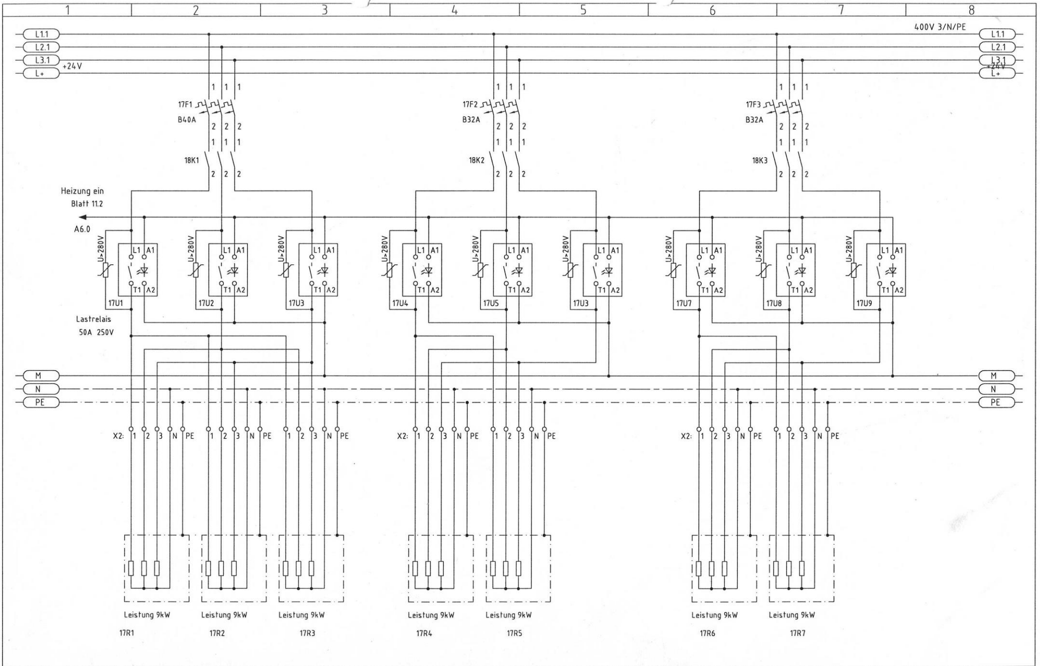
Heizung Behälter 1 7x9kW
