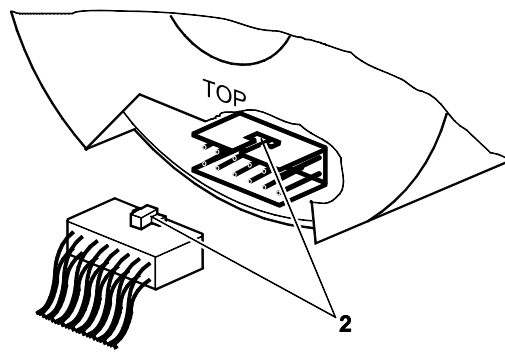
Bild 16 Elektrischer Geberanschluss
