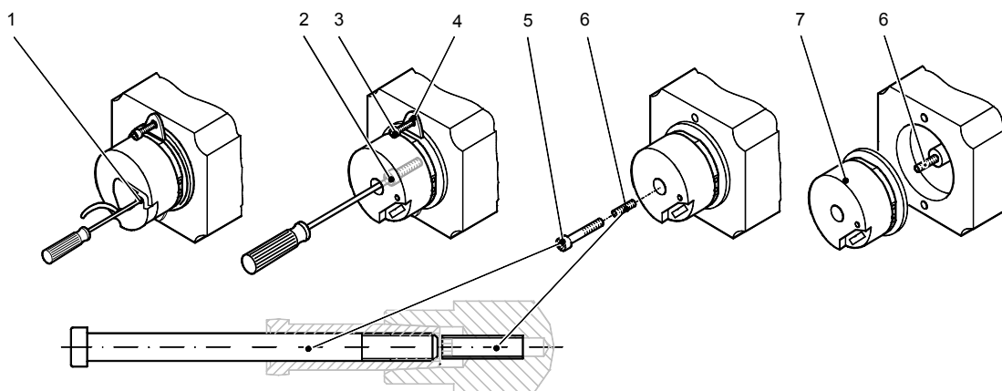
Bild 5 Abdrücken des Gebers mit Gewindestift und Schraube oder Sonderschraube
