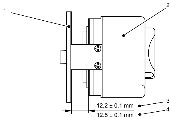
Bild 7 Montage bei Motor 1FT603.-04
