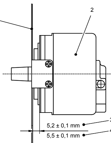
Bild 11 Montage bei Motoren
