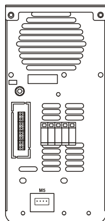
FIG. 3A (Denominazione dei componenti - Dimensioni / Component names - Sizes)
