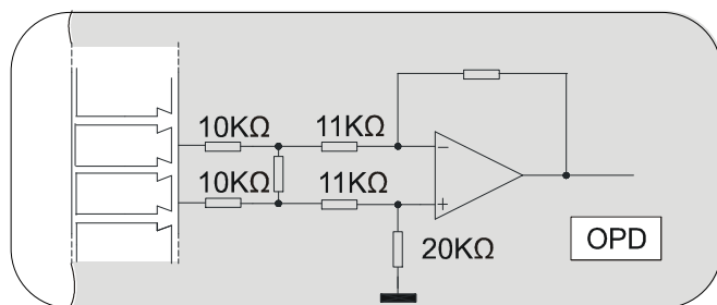
FIG. 13 (Ingresso analogico configurabile / Configurable analog input)
