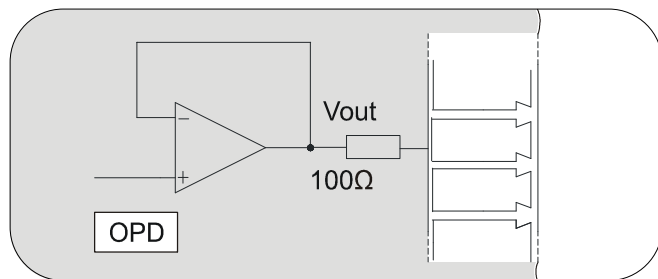
FIG. 15 (Uscita analogica configurabile / Configurable analog output)
